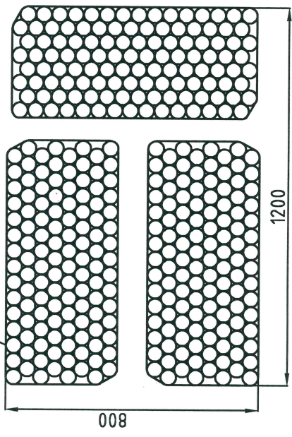
Нечетный слой
